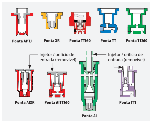
Figura 4. Desenho de corte de seções das pontas de pulverização APTJ, XR, TT, TTJ60, AIXR, AITTJ60, AI, TTI60.
