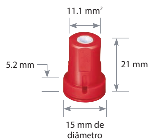
AITXB ConeJet
