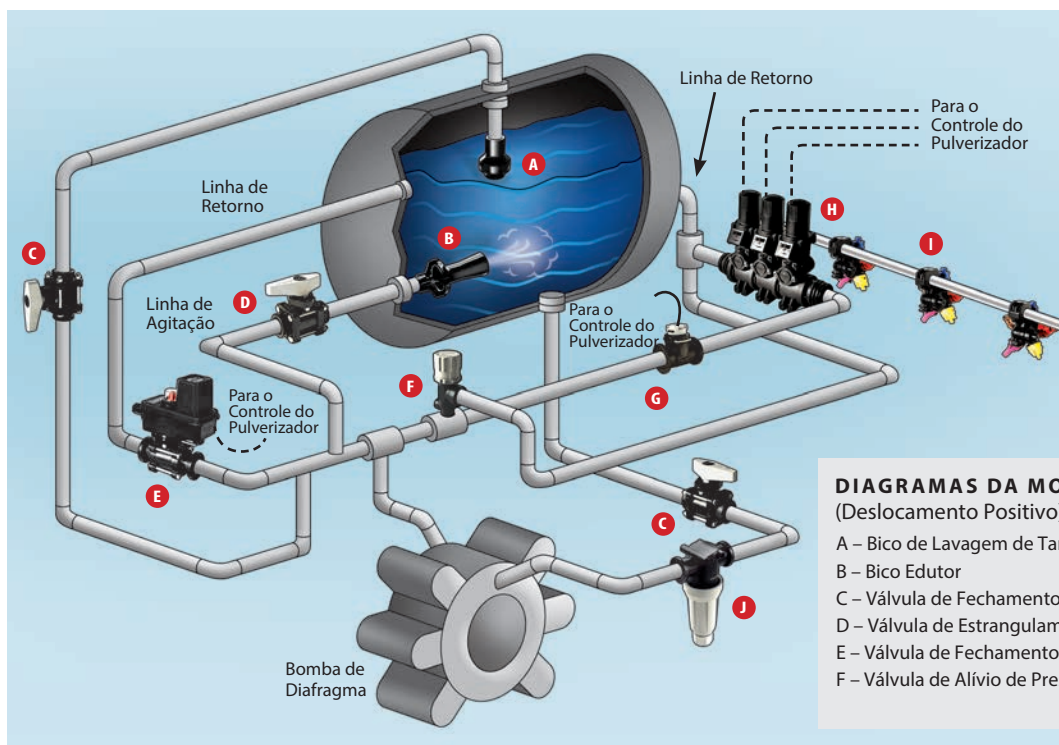
DIAGRAMAS DA MONTAGEM DE DUAS VIAS (Deslocamento Positivo) A – Bico de Lavagem de Tanque G – Fluxômetro B – Bico Edutor H – Comando Manifold de 2 Vias C – Válvula de Fechamento Manual I – Corpos de Bico e Pontas de Pulverização D – Válvula de Estrangulamento J – Filtro de Linha E – Válvula de Fechamento Elétrica F – Válvula de Alívio de Pressão
